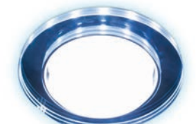
G214 CL/CH/CLD D 120 мм H 39 мм A 87 мм LED лента 3W COLD + GX53 LED max 12W
